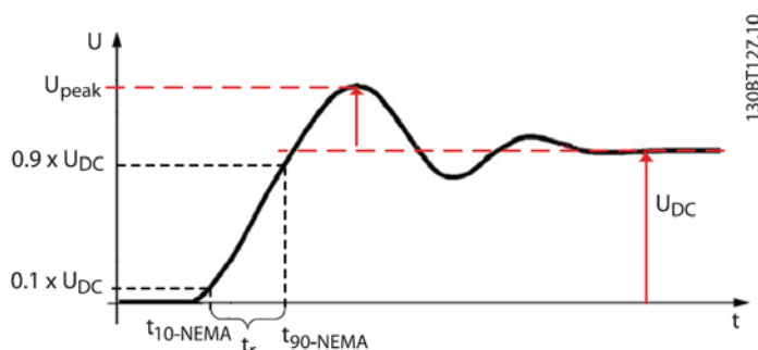
Рис. 3.3 Стандарт NEMA
