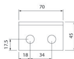
Рис. 5.16 Комплект L-образных клемм 130B3138
