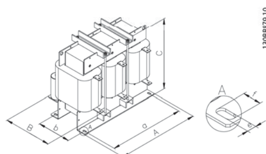
Рис.5.7 Фильтр IP00 напольный
