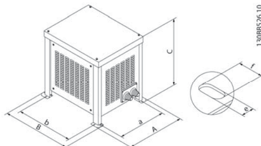
Рис.5.6 Фильтр IP23 напольный
