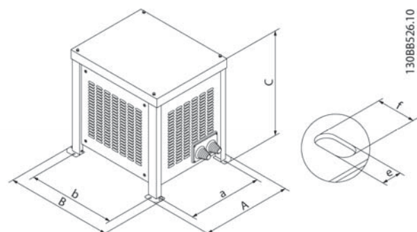
Рис. 5.12 Фильтр IP23 напольный
